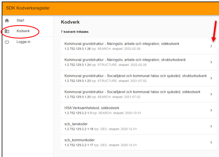
Bild 2: SDK Kodverksregister
